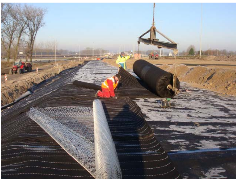
Foto: Bij 11: Aanbrengen drainagemat en geogrids.
